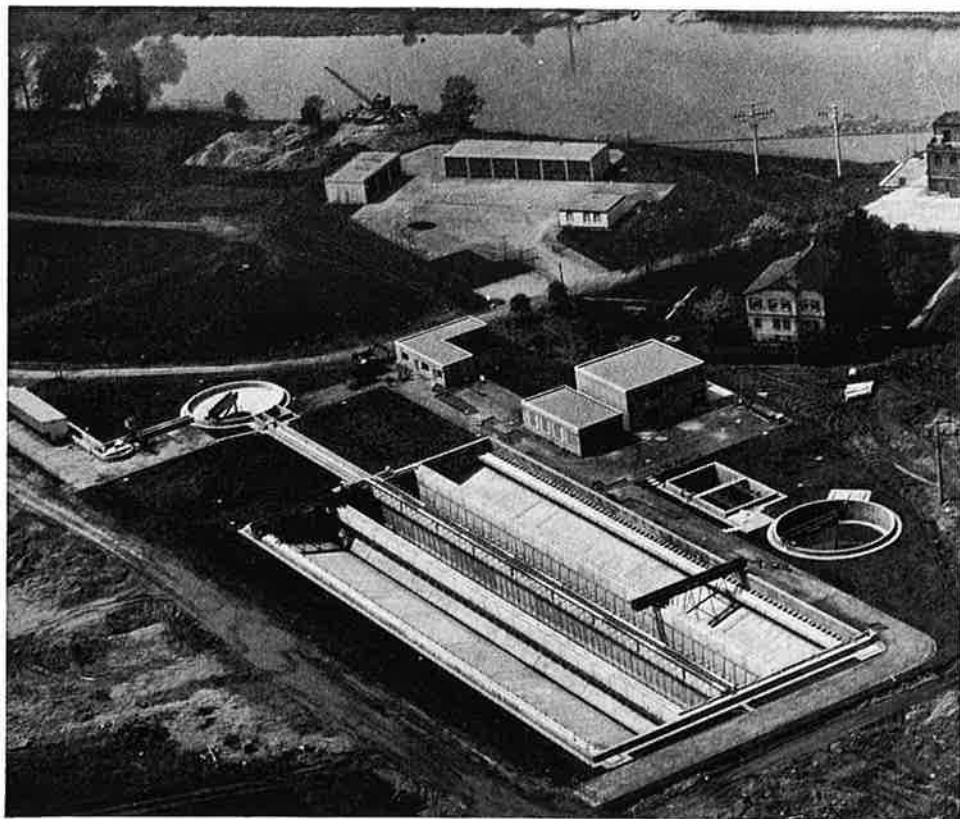
WIBAU Kläranlage Rottenburg/Neckar Luftbild freigegeben unter Nr. 389/75 Reg. Präs. Darmstadt
